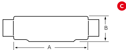
Corps de conduits et couvercles, modèle C, Forme 7, en fer
