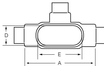
Corps de conduits et couvercles, modèle T, Marque 9, en aluminium
